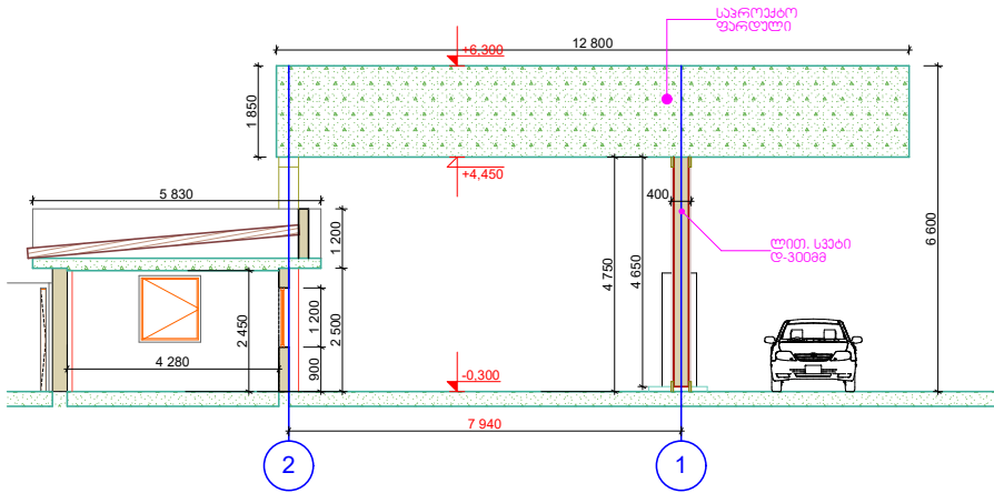
არს.ჭრილი 1-1
